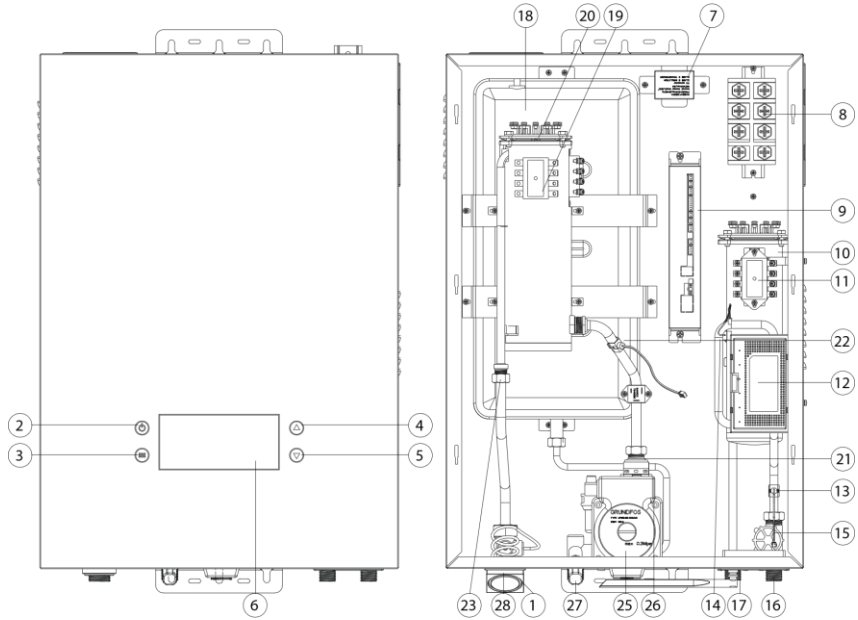
Рис. 1. Конструкция изделия
